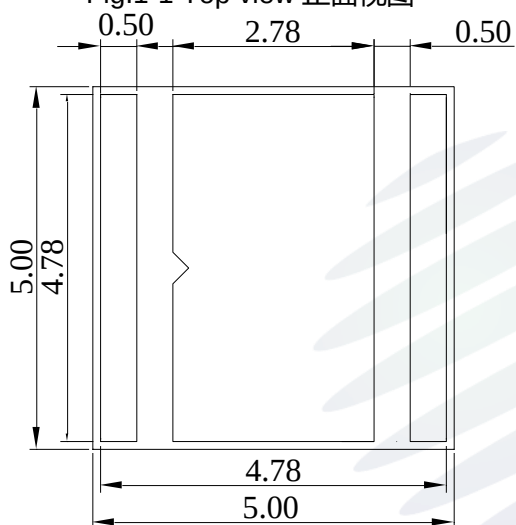
Fig.1-3 Bottom view 背面视图
