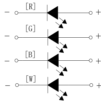
Fig.1-4 Polarity 极性
