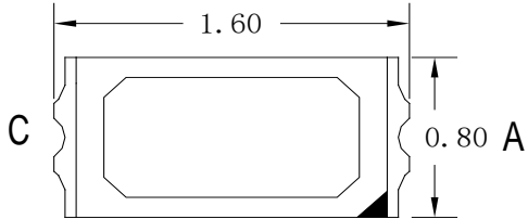
Fig. 1-1 Top View 正面视图
