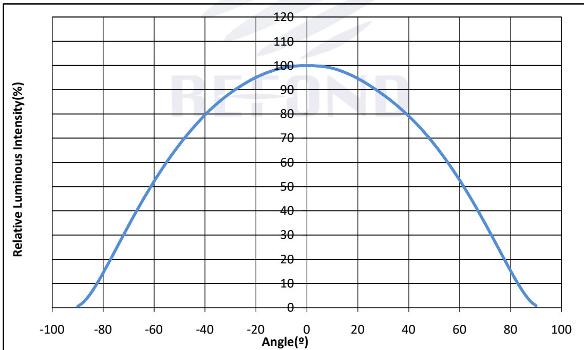
Fig. 1-12 Radiation diagram 辐射特性曲线
