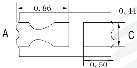
Fig. 1-3 BottomView 背面视图
