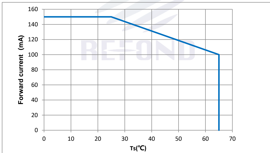
Fig 1-9 Ts Temperature Vs Forward Current 管脚温度与正向电流特性曲线
