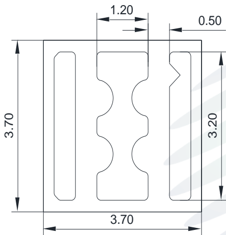
Fig.1-1 Top view 正面视图
