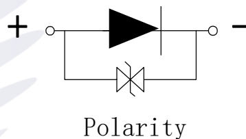
Fig.1-4 Polarity 极性
