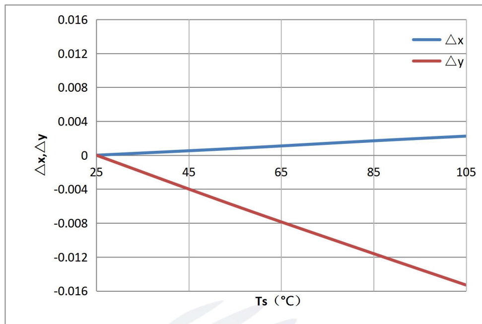
Fig 1-13 \Delta CIE_x, CIE_y vs Temperature xy与温度特性曲线
