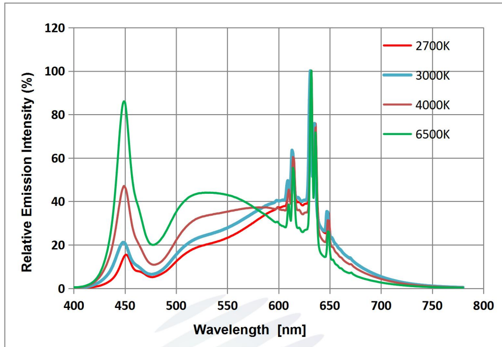
Fig 1-15 Spectrum Distribution光譜分布特性曲线
