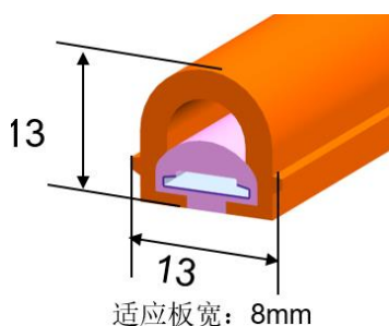
Product section 产品截面尺寸(参考外形尺寸)
