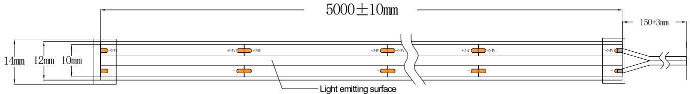
Fig.1-2 Top View 正面视图
