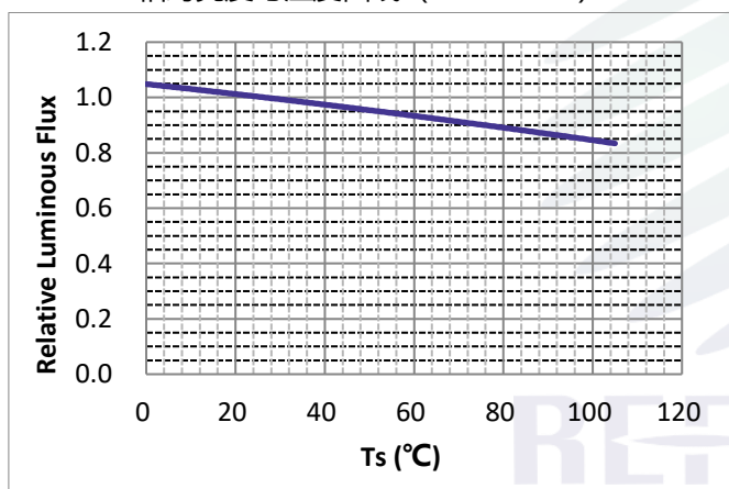
Relative luminous flux vs. Ts temperature 相对亮度与温度曲线 (IF=800mA)
