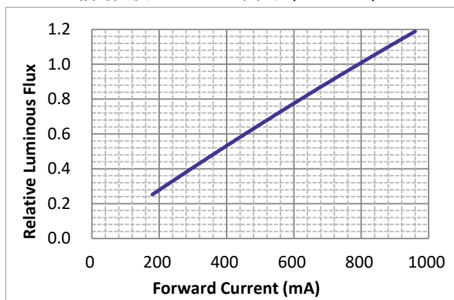
Relative luminous flux vs. forward current 相对亮度与正向电压曲线 (Ts=25°C)
