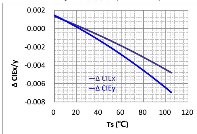
ΔCIE-x/y vs. Ts temperature ΔCIE-x/y 与温度曲线 (IF=800mA)
