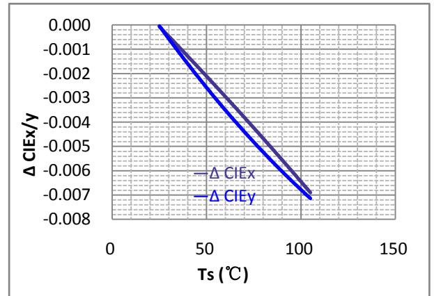
ΔCIE-x/y vs. Ts temperature ΔCIE-x/y 与温度曲线 (IF=65mA)
