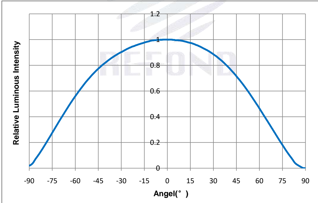
Fig 1-8 Radiation diagram 辐射特性曲线
