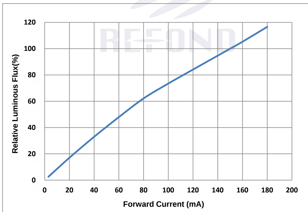
Fig. 1-8 Forward Current Vs Relative Intensity 正向电流与相对光通量特性曲线
