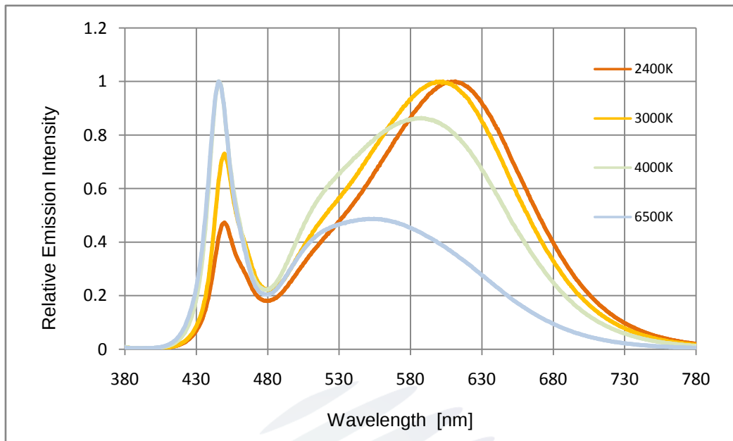
Fig 1-13 Spectrum Distribution光譜分布特性曲线
