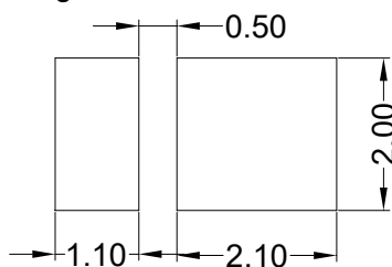
Fig.1-3 Bottom view 背面视图
