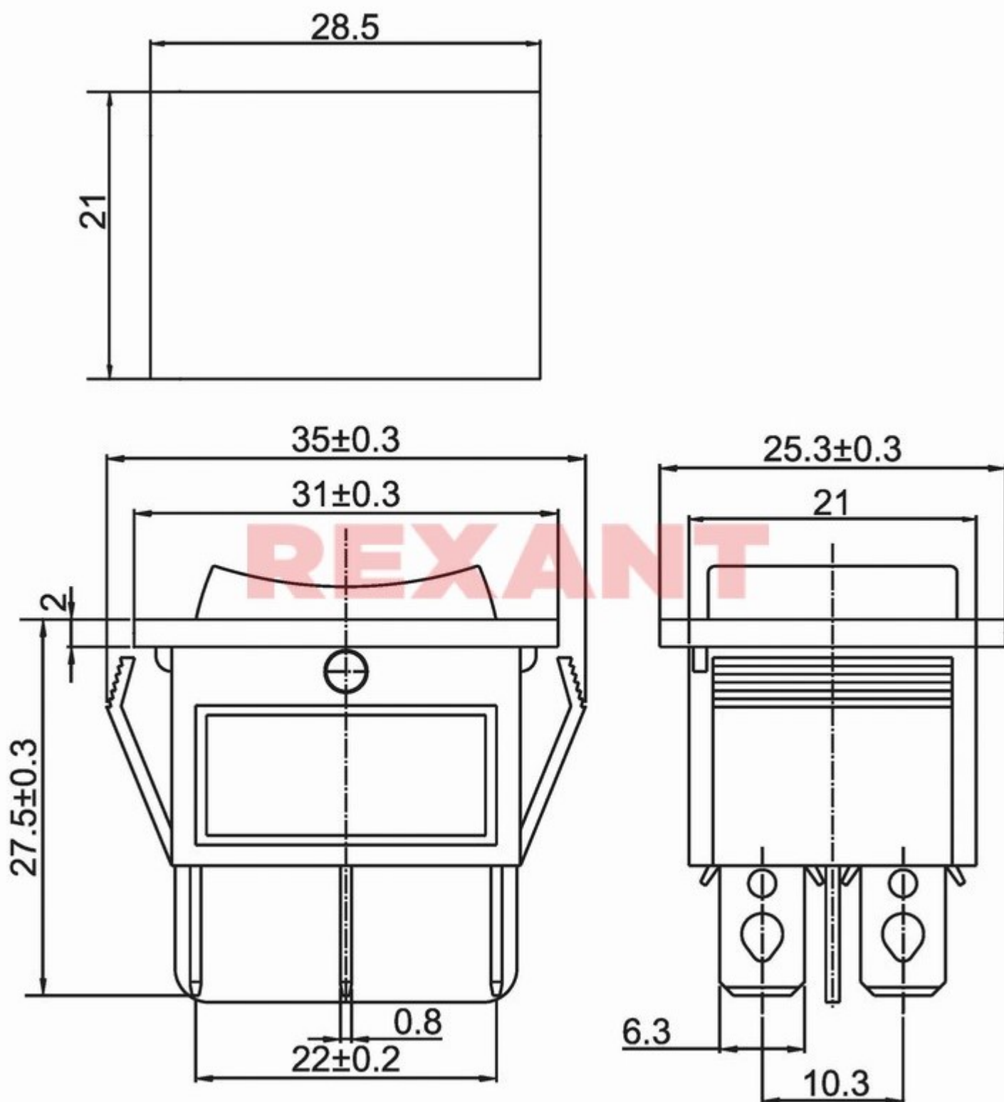
Выключатель клавишный 250V 15A (6c) ON-OFF-ON черный с нейтралью REXANT
