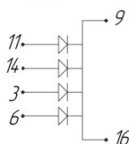
542НД2, К542НД2
