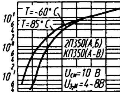
Проходные характеристики
