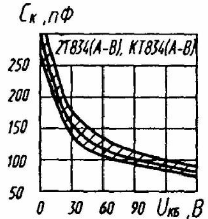
Зона возможных положений зависимости емкости коллекторного перехода от напряжения коллектор—база
