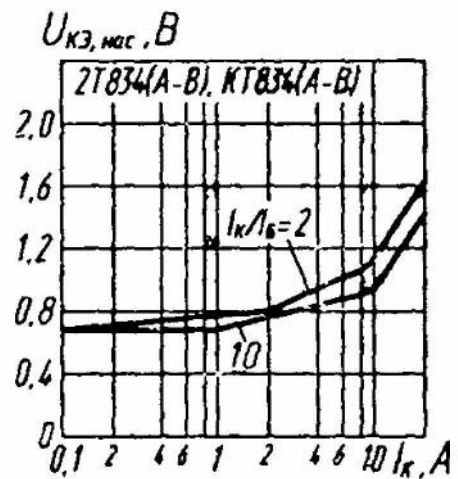
Зависимости напряжения насыщения коллектор—эмиттер от тока коллектора
