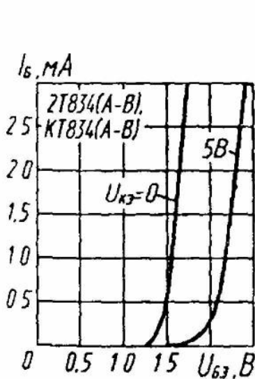
Входные характеристики
