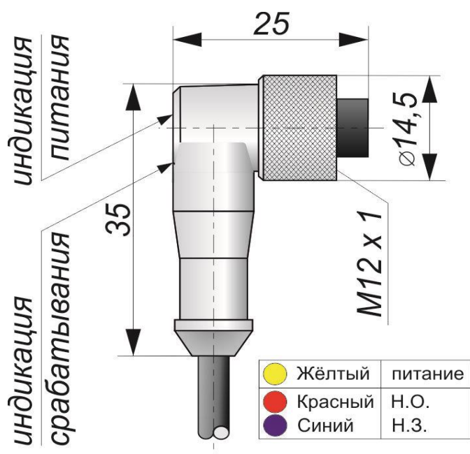
Габаритный чертеж
