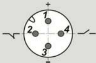
Цоколевка разъема
