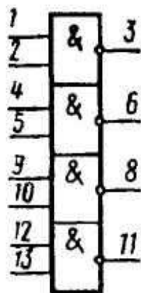
Условное графическое обозначение К155ЛА12, КМ155ЛА12
