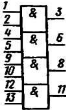
Условное графическое обозначение К555ЛИ1, КМ555ЛИ1
