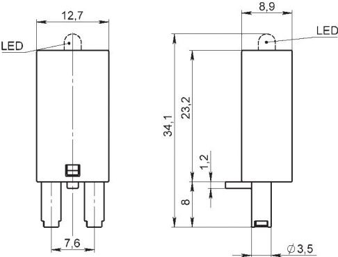
Рисунок 1 – Габаритные, установочные присоединительные размеры модулей
