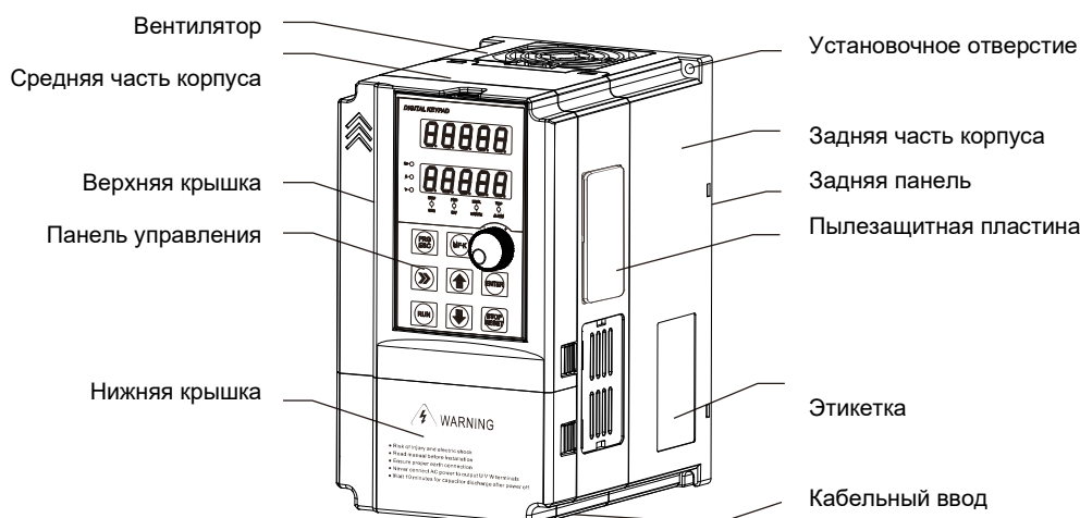
Рис 2-2 Внешний вид
