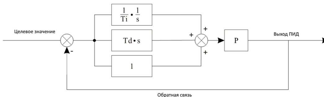
Рис. 5-25 Блок-схема ПИД-регулирования.
