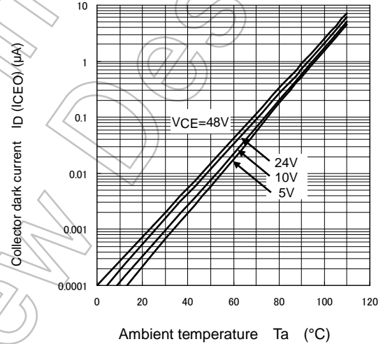
I_{CE0} - T_a
