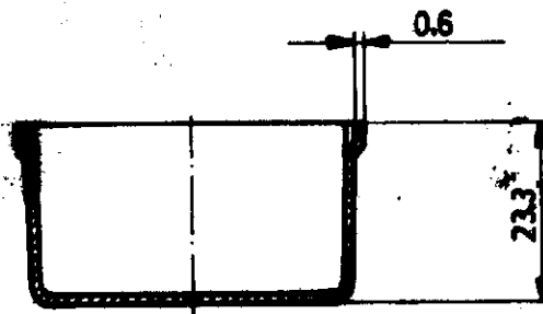
SCHNITT A-A
