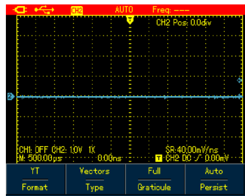
Рисунок 6-14. Настройка изображения осциллограммы
