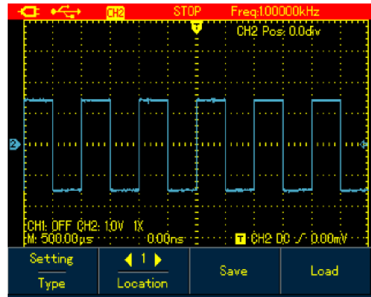
Рисунок 6-24. Воспроизведение записанной осциллограммы
