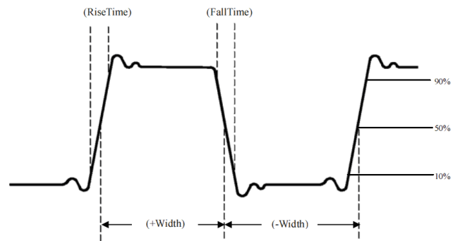
Рисунок 6-21. Измеряемые параметры времени
