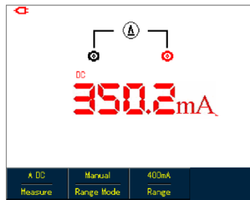
Рисунок 5-15. Измерение постоянного тока от 40 до 400 мА (UTD1000DL)
