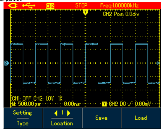
Рисунок 6-25. Меню сохранения настроек и осциллограмм
