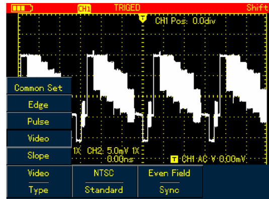
Рисунок 6-11. Запуск по видеосигналу
