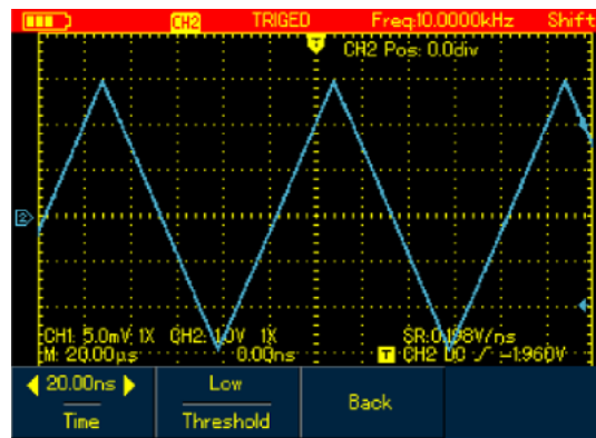
Рисунок 6-13. Запуск по наклону фронта (страница 2)
