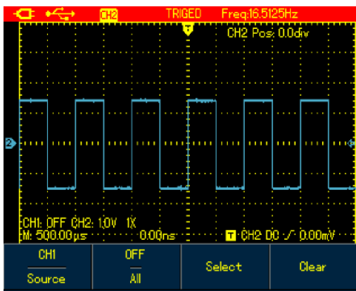
Рисунок 6-15(б). Меню автоматических измерений модели UTD1000DL
