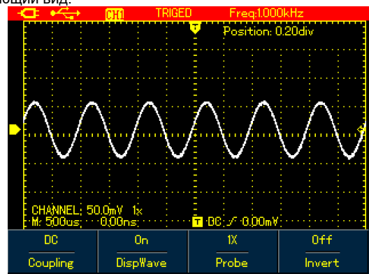
Рисунок 6-1(a). Меню настройки канала (UTD1000CL)
