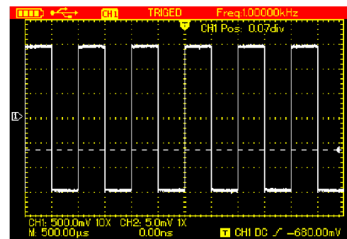
Рисунок 4-8. Настройка уровня запуска
