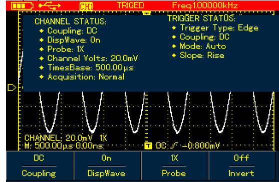
Рисунок 4-15(a). Информация о состоянии осциллографа UTD1000CL
