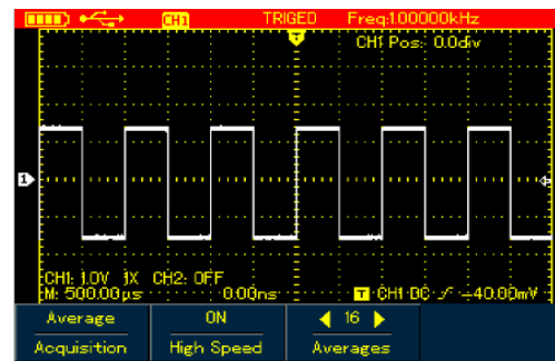
Рисунок 4-19. Сглаживание в режиме усреднения по 16 наборам данных
