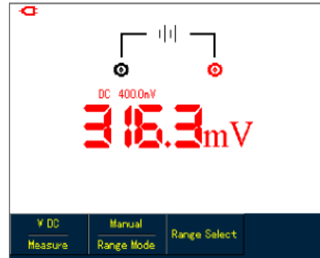
Рисунок 5-23. Ручной выбор предела измерения
