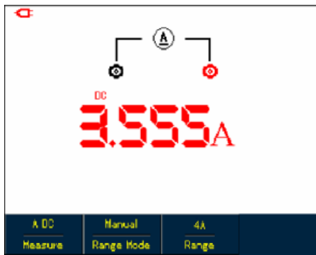
Рисунок 5-16. Измерение постоянного тока более 400 мА (UTD1000DL)
