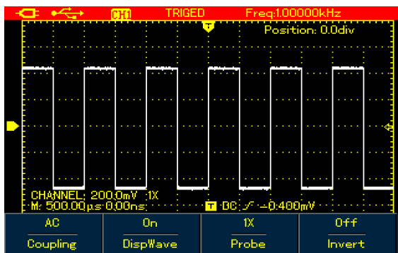
Рисунок 4-22(a). Работа в режиме связи по переменному току в модели UTD1000CL
