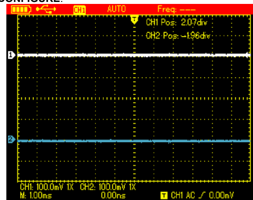
Рисунок 4-3. Отключение меню
