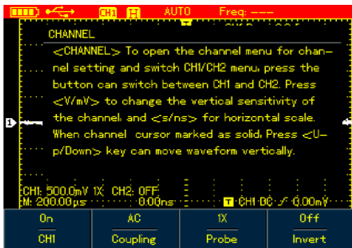
Рисунок 4-13. Встроенная справка
