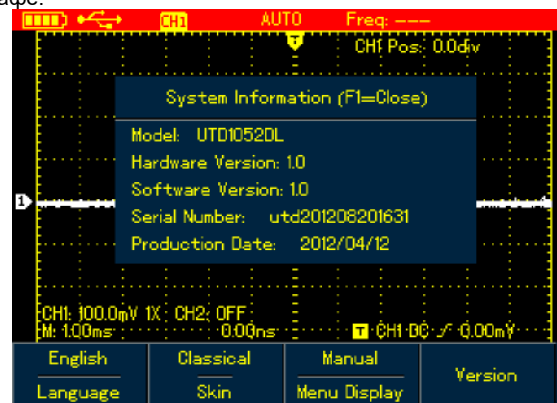
Рисунок 4-16. Системная информация
