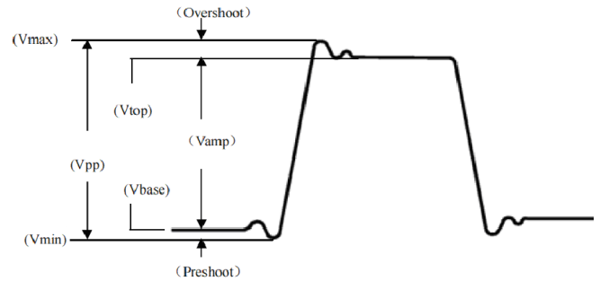
Рисунок 6-20. Измеряемые параметры напряжения
