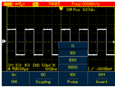
Рисунок 4-4. Установка коэффициента ослабления щупа
