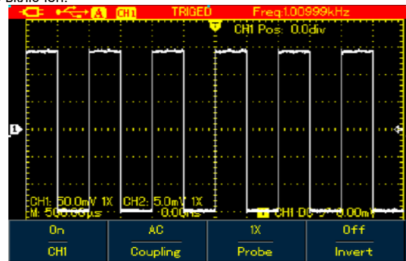
Рисунок 4-11. Частотомер пускового сигнала в модели UTD1000CL
