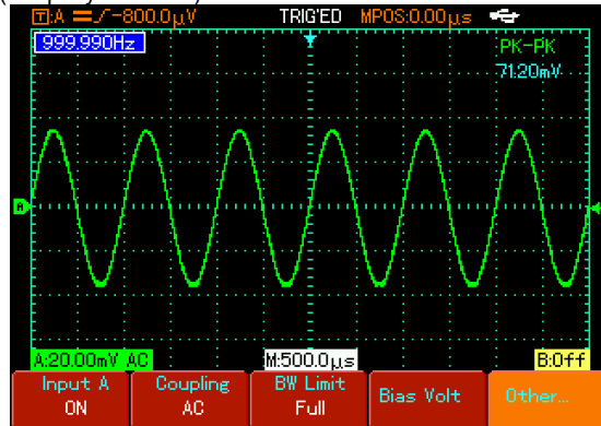
Рисунок 4-25. Изменение параметров переменной составляющей сигнала
