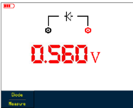
Рисунок 5-2. Проверка диодов
