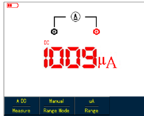
Рисунок 5-13. Измерение постоянного тока до 1 мА (UTD1000DL)
