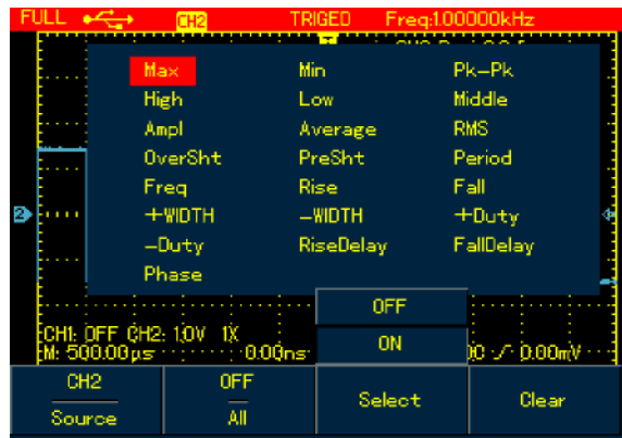
Рисунок 4-18(б). Измерение выборочного набора параметров в осциллографе UTD1000DL
