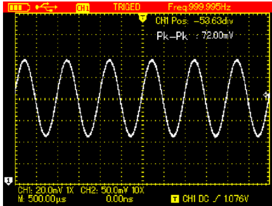
Рисунок 4-24(а). Осциллограмма сигнала с постоянной составляющей (модель UTD1000CL)
