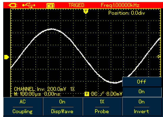
Рисунок 4-23(a). Обращенная осциллограмма (модель UTD1000CL)
