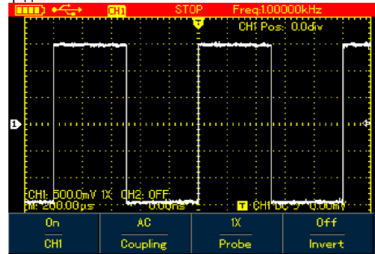
Рисунок 4-10. Остановка сбора данных
