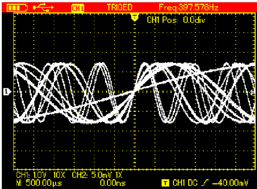
Рисунок 4-21. Послесвечение дисплея, установленное на 3 с
