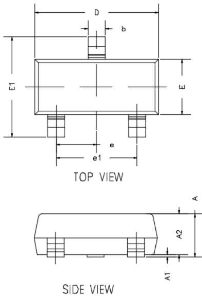
SOT-23
