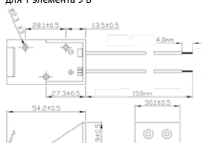
GSN-9V-1A для 1 элемента 9 В
