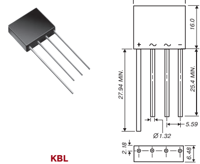
KBL
