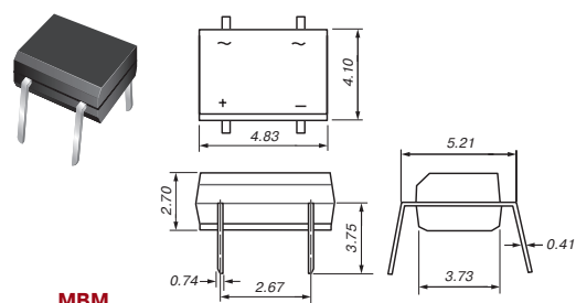
MBM
