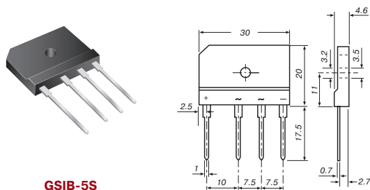
GSIB-5S
